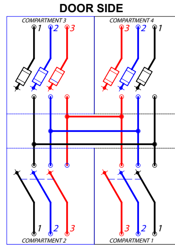
PMH-9 DOOR SIDE
